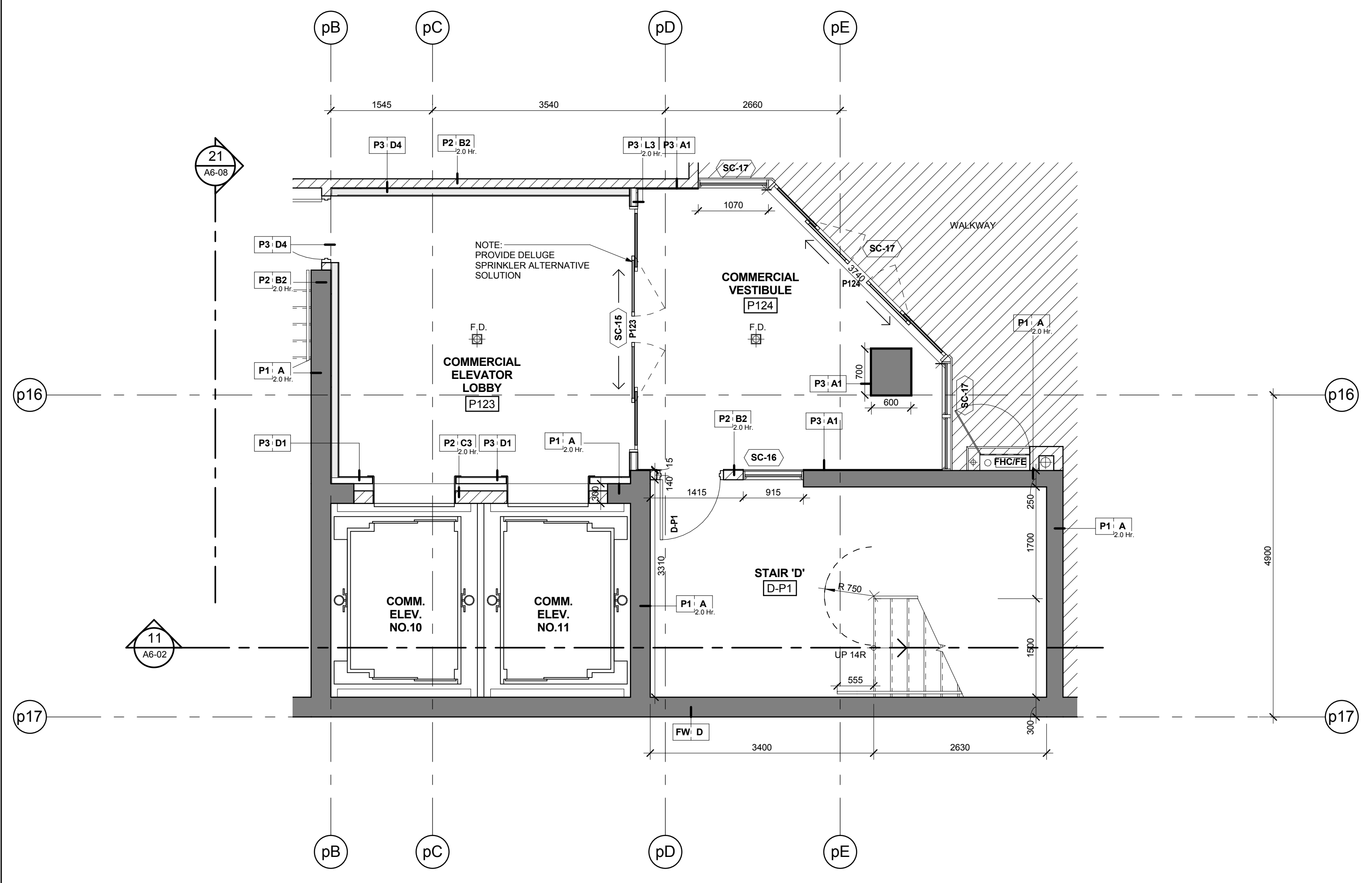
Stair 'D' - Stair Plan - Level P1 8 Scale: 1 : 50 A6-02
