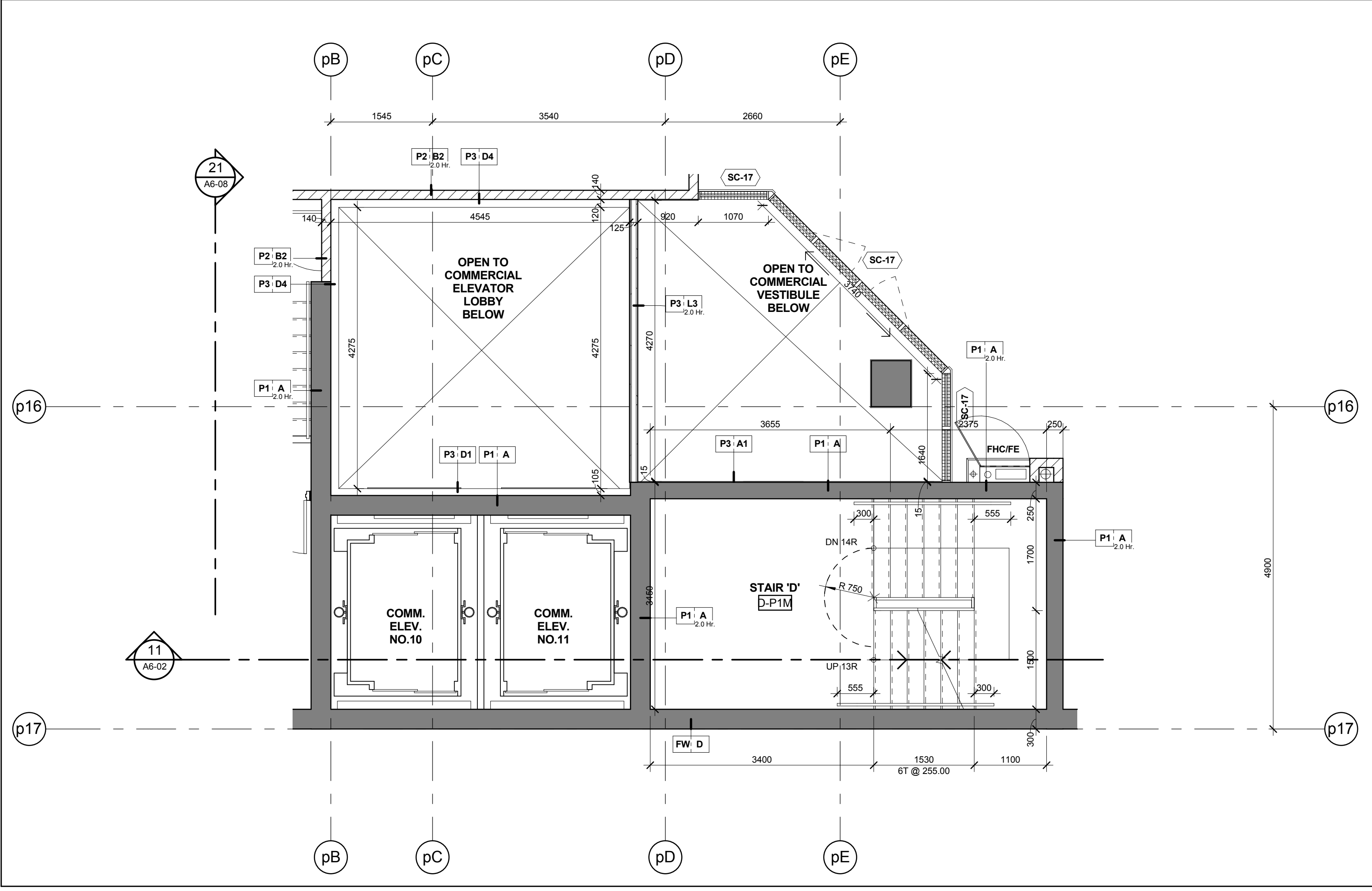
Stair 'D' - Stair Plan - Level P1 Mezzanine 9 Scale: 1 : 50 A6-02
