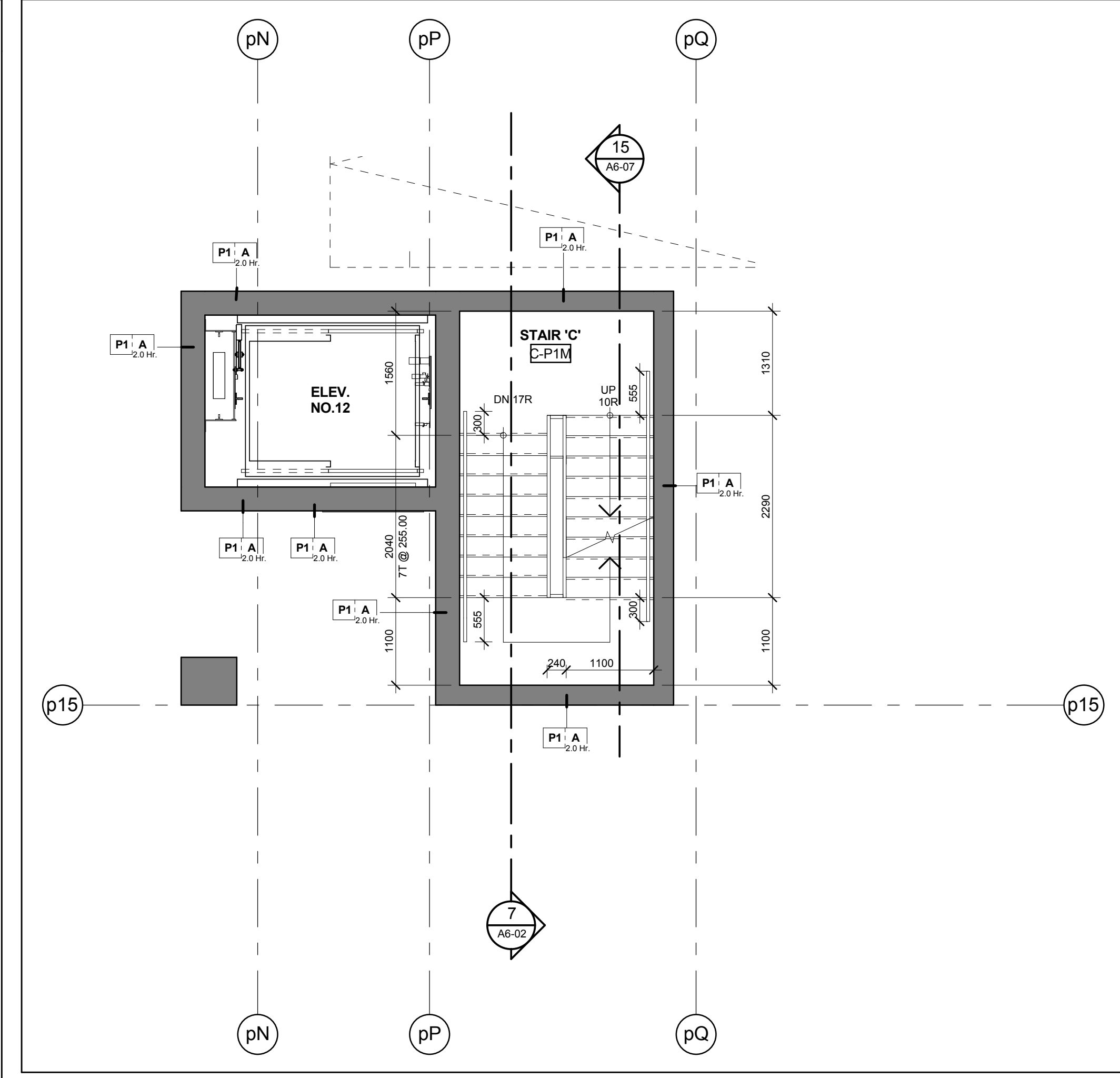
Stair 'C' - Stair Plan - Level P1 Mezzanine 5 Scale: 1 : 50 A6-02
