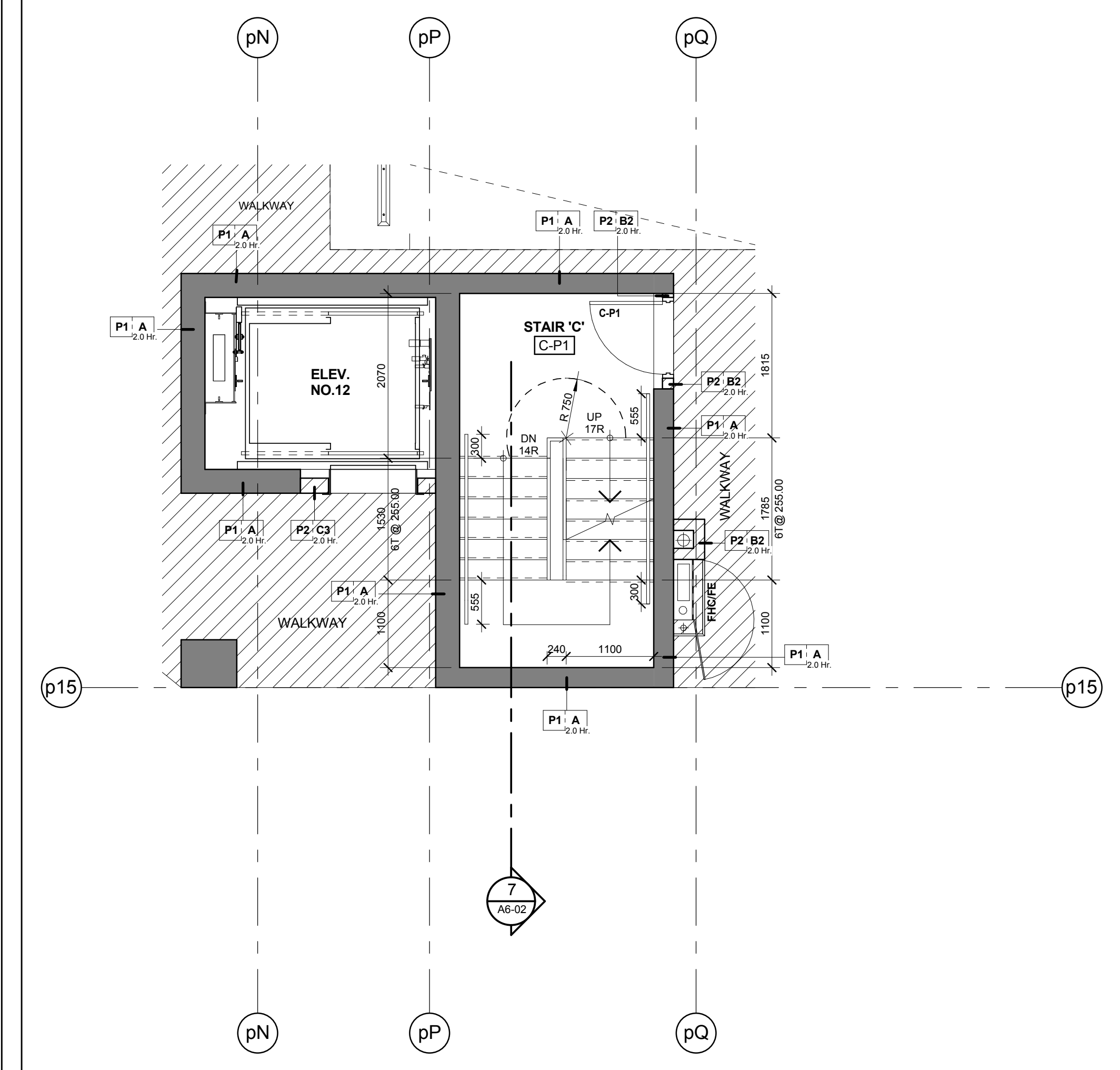
Stair 'C' - Stair Plan - Level P1 4 Scale: 1 : 50 A6-02
