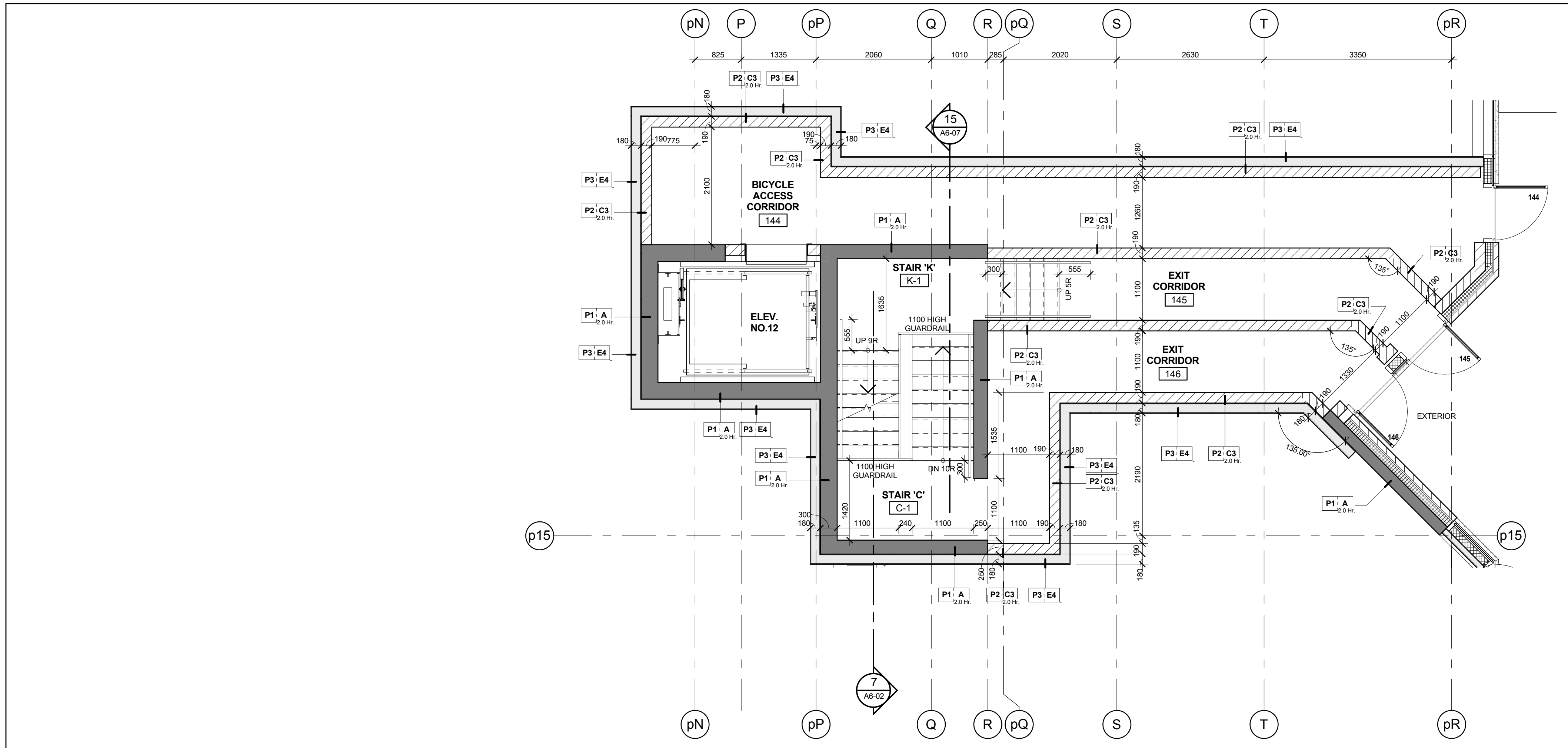
Stair 'C' - Stair Plan - Level 1 6 Scale: 1 : 50 A6-02
