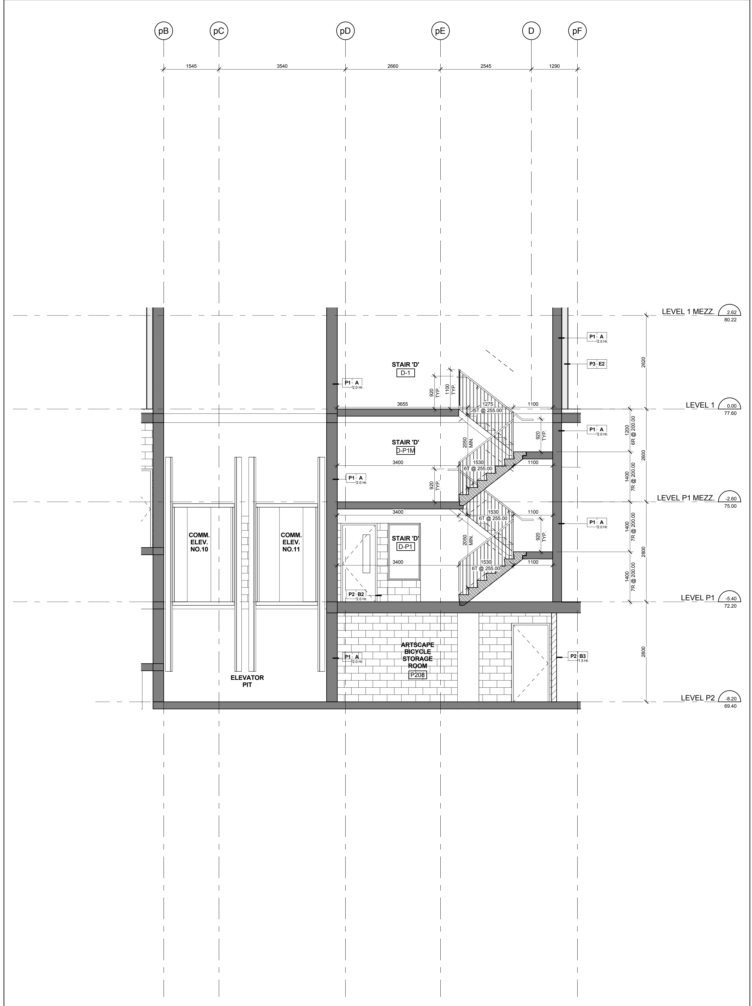
Stair 'D' - Stair Section - Levels P2 - 1 Mezzanine 11 Scale: 1 : 50 A6-02
